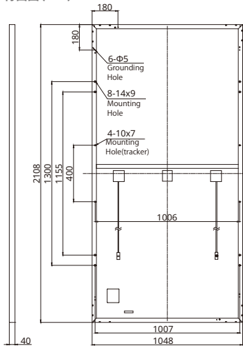
背面図 (mm)
