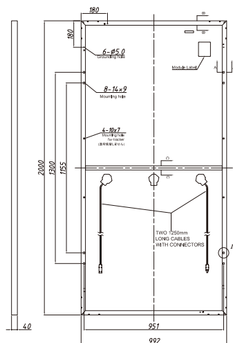
背面図 (mm)
