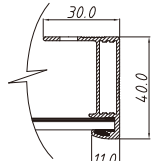
アルミニウムフレーム C-C
