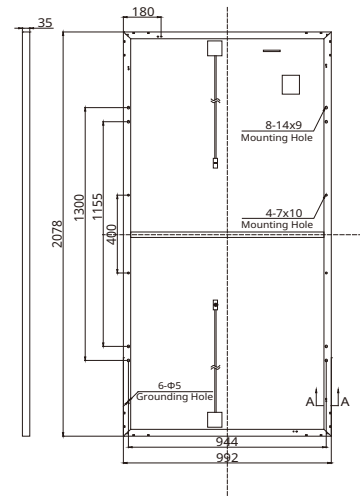
背面図 (mm)
