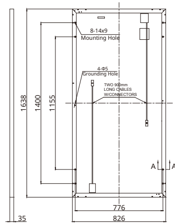
背面図 (mm)
