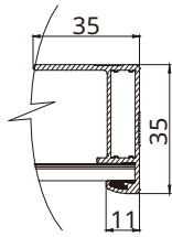
フレーム断面図 A-A
