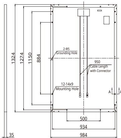
背面図 (mm)
