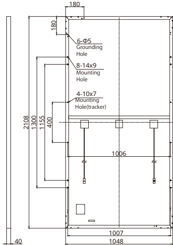
背面図 (mm)
