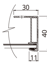
フレーム断面図 A-A
