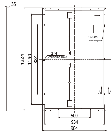
背面図 (mm)
