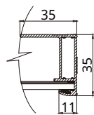
フレーム断面図 A-A
