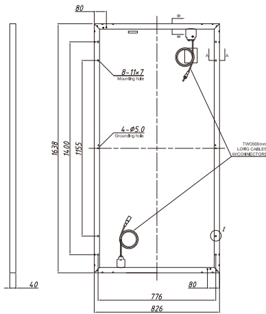
背面図 (mm)
